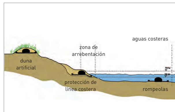
Estabilización de costas con distintas posibilidades de utilización de SoilTain CP y manto anti-socavación paralelos a la línea costera
