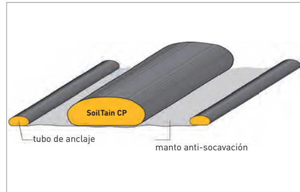
Ilustración de un tubo SoilTain como rompeolas con manto anti-socavación provisto de tubos de anclaje
