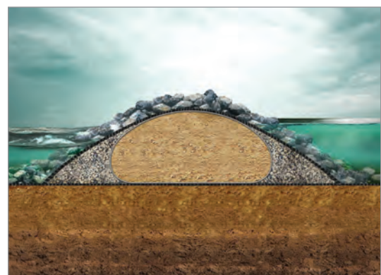
Rompeolas sumergido Protección frente a la erosión Incrementa la deposición de arena
